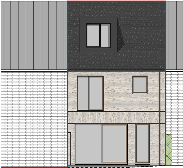
achtergevel
